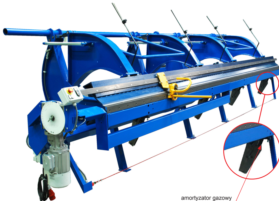
amortyzator gazowy
