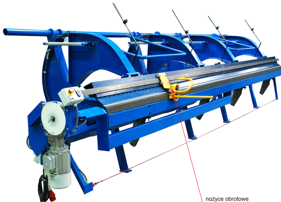
nożyce obrotowe
