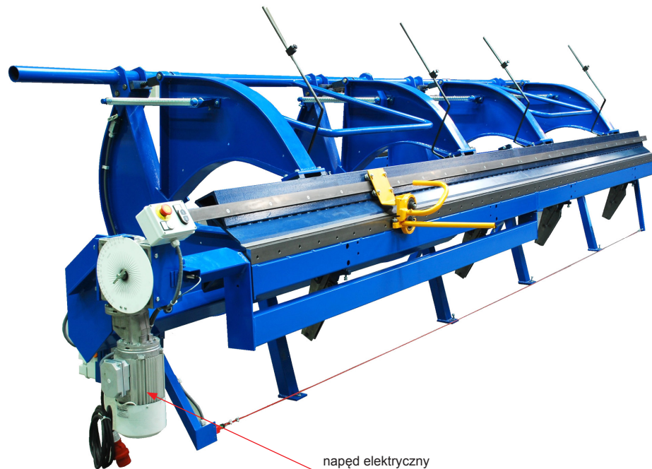
napęd elektryczny
