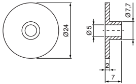
Podkładka gumowa
