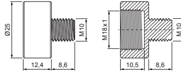
Część górna
