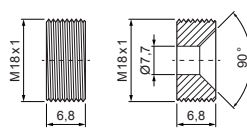
Część dolna
